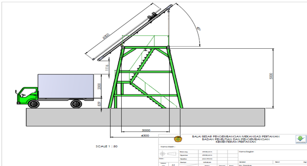
Gambar 2. Desain mesin core sampler tebu (tampak samping)
